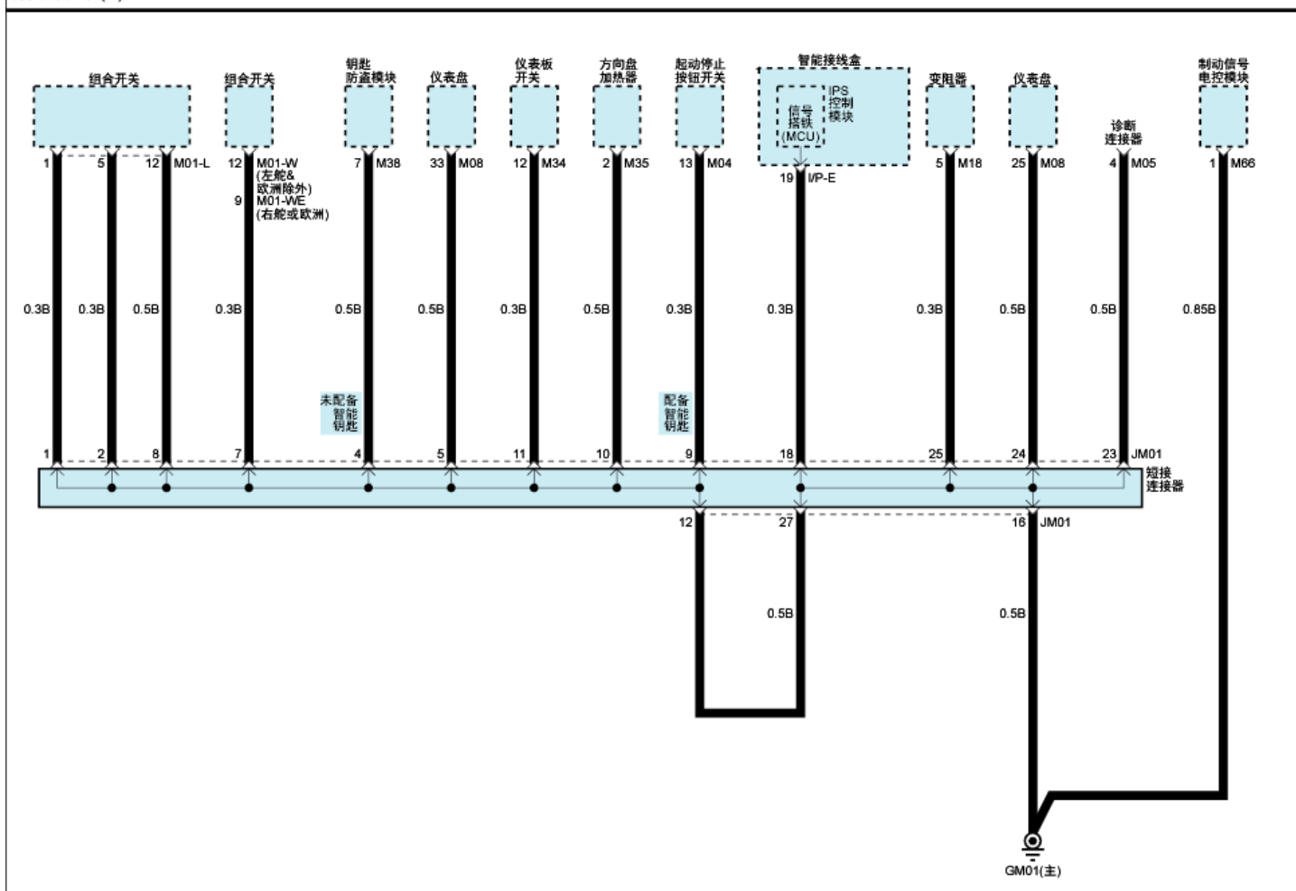
搭铁分布(1)
